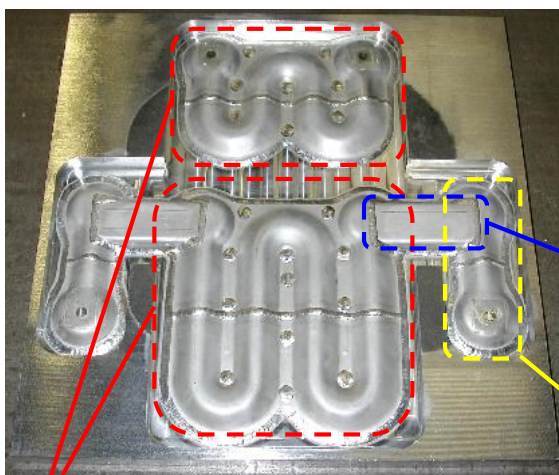
1パス プレートコイル
